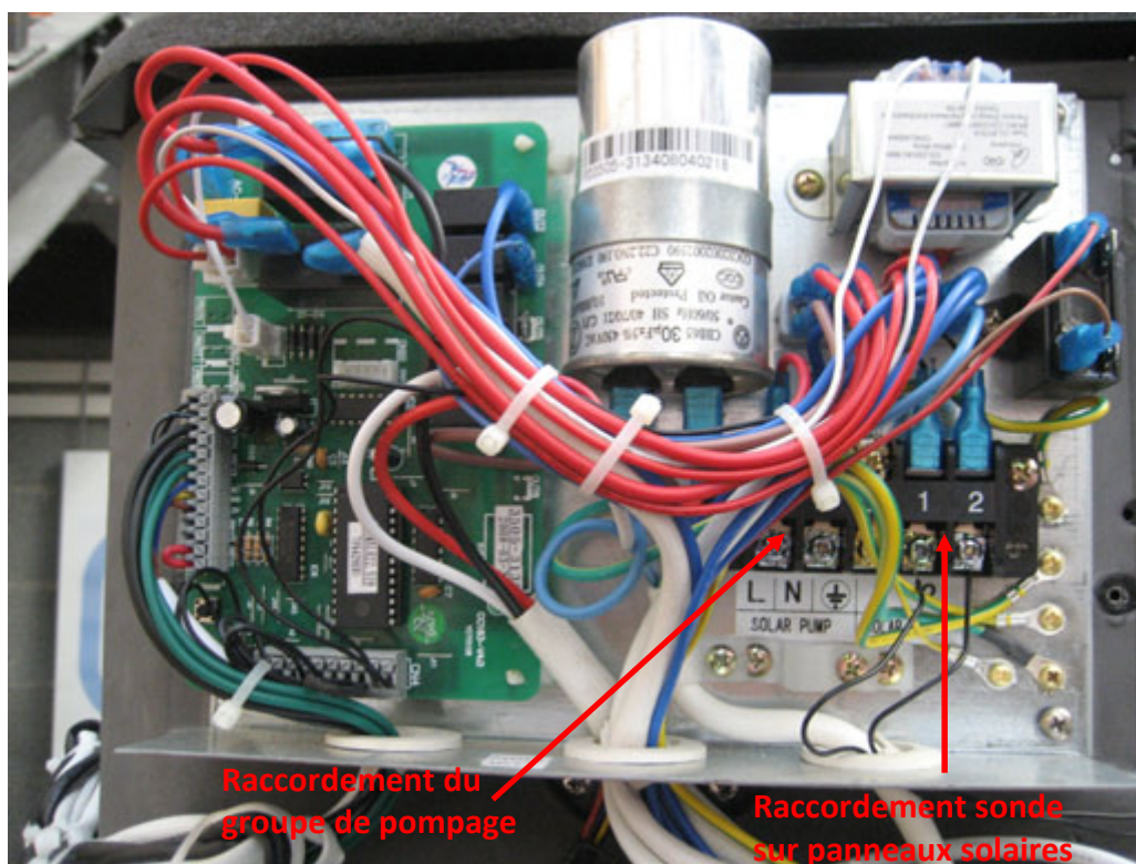
Modèle équipé de la régulation solaire dans la PAC-ECS (décembre 2009) Fig. 1
